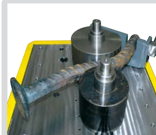
Kör keresztmetszet anyagok hajlításához 40 mm átmérőig
